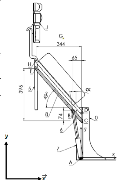
figure 14 - Position où l'effort du vérin est maximum.
