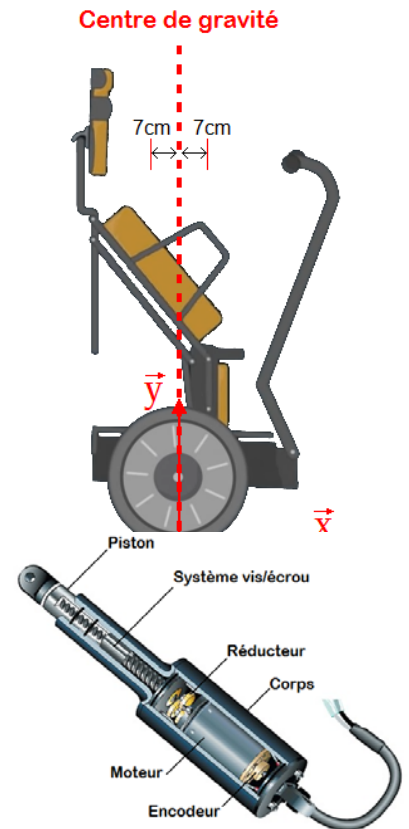
figure 5 - Vérin électrique.
